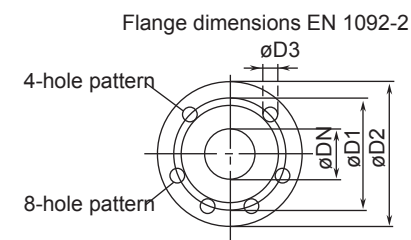
Flange dimensions in acc.with DIN EN 1092-2
